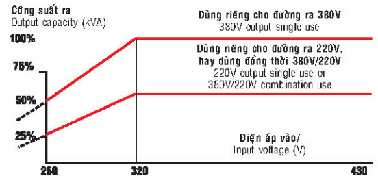
Đồ thị giới hạn công suất ra ở các mức điện áp vào The output capacity limit chart at input voltage level
